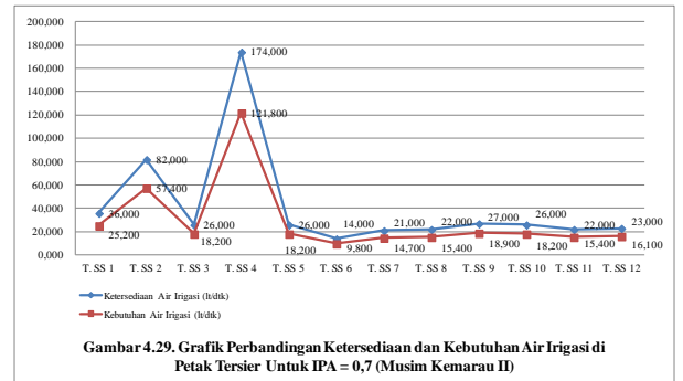
Gambar 4.29. Grafik Perbandingan Ketersediaan dan Kebutuhan Air Irigasi di Petak Tersier Untuk IPA = 0,7 (Musim Kemarau II)
